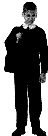
4 Jack
