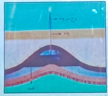
لایه‌های رسوبی
