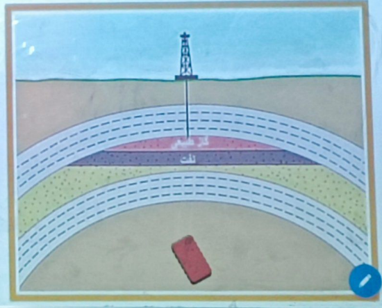
لایه‌های رسوبی
