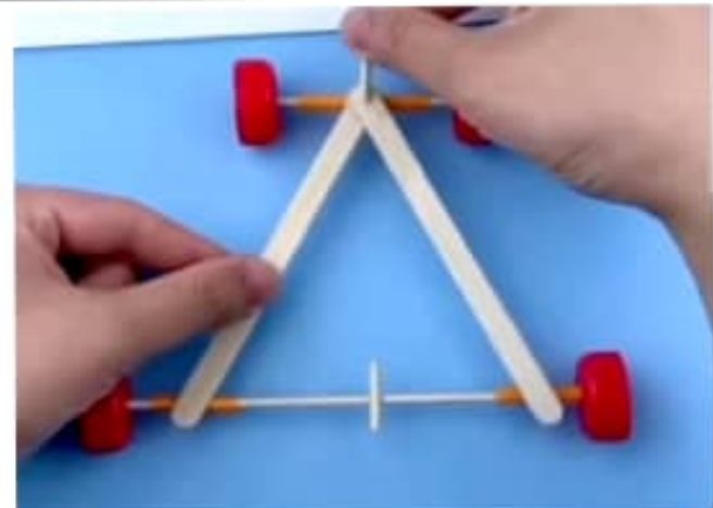
۶_ بر گرداندن چوب های بستنی و چسباندن دو قطعه سیخ چوبی کوچک (۲ تا ۳ سانتی متر) روی ماشین مطابق تصویر
