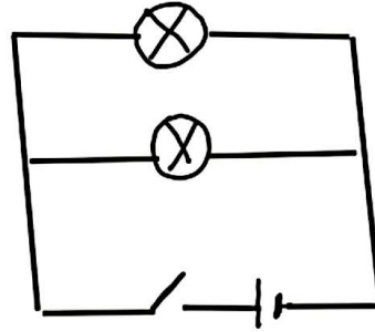
مدار موازی
